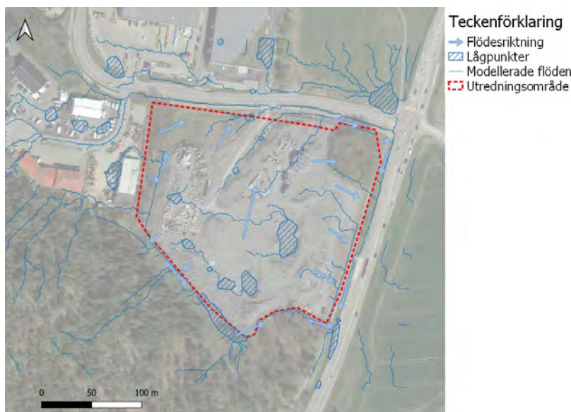
Figur 32. Befintlig ytavrinning inom planområdet samt flöden och närliggande lågpunkter.
