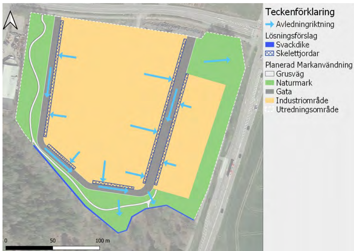
Figur 33. Illustration av exempel på placering för dagvattenlösningar och hur dagvatten bör avledas. (Tyréns, 2022b)
